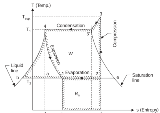
Fig. 14.11. T-s diagram.
