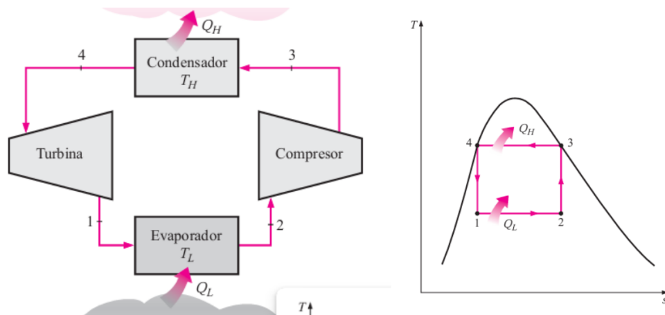
Figura A.4: Ciclo Carnot inverso.
